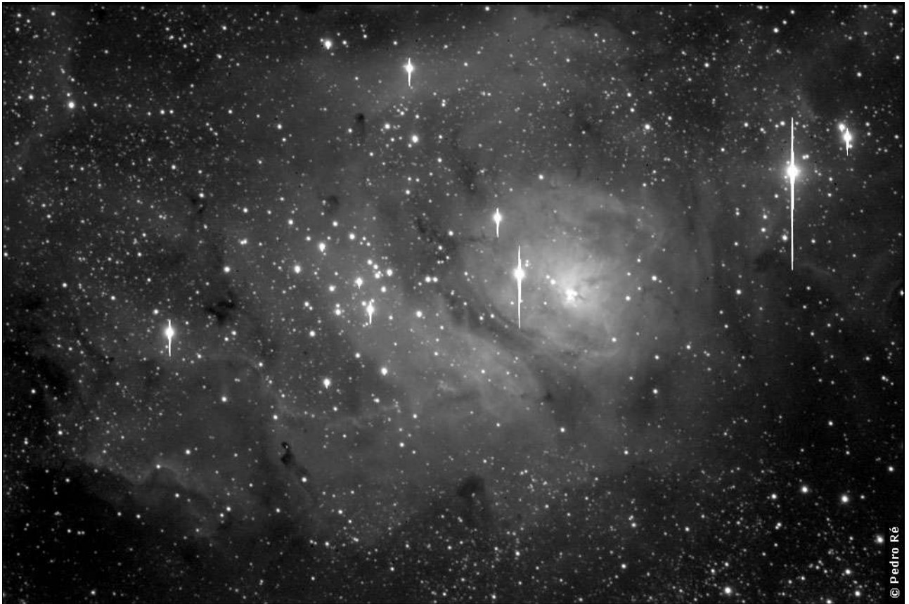
Figura 13- M8, Montagem EM-200, FS128 F/8.1, SBIG ST-8E (auto-guiagem), 15 min, 5x3 min (soma), log scaling. Pedro Ré (2003).
