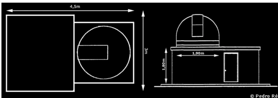
Figura 1- Alçado superior e lateral do observatório.
